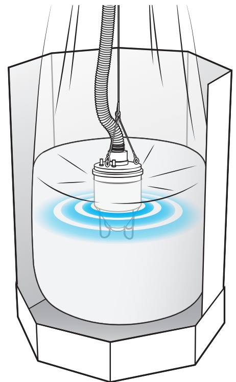
Têtes d'aspiration vibrantes
