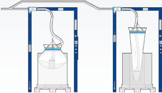
Doppelstation mit Weitschaltung
