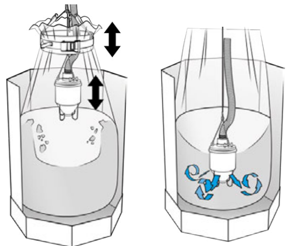
Fluidisierung
